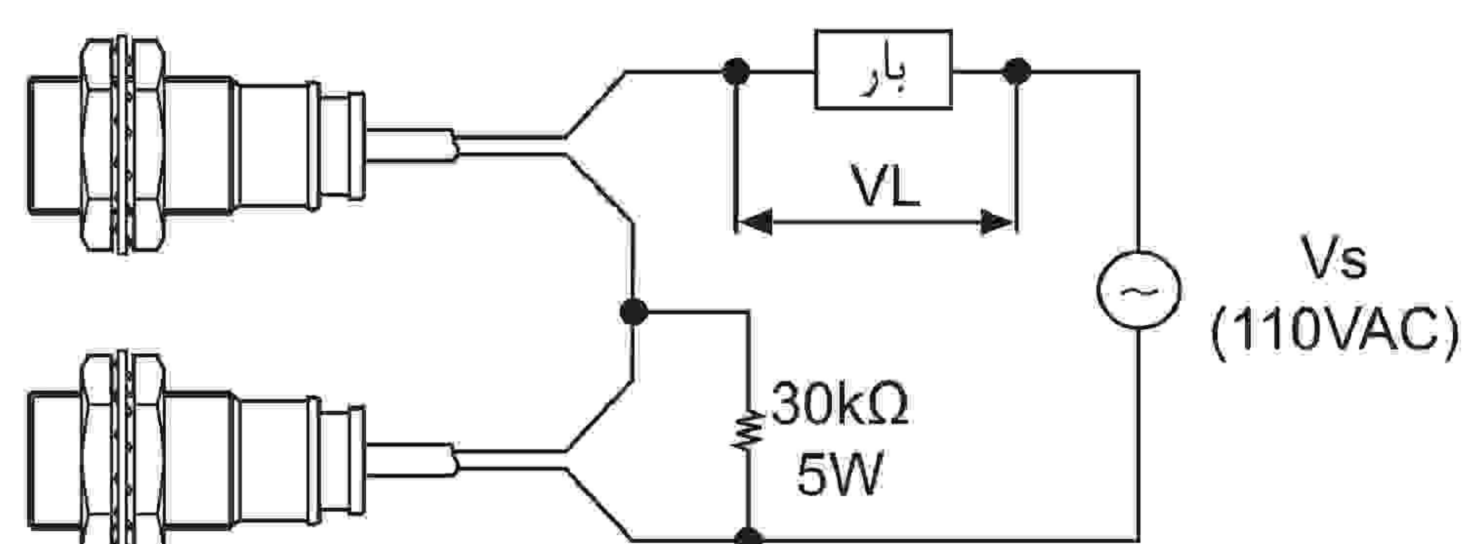
روش اتصال مقاومت تخلیه (شکل ۳)
