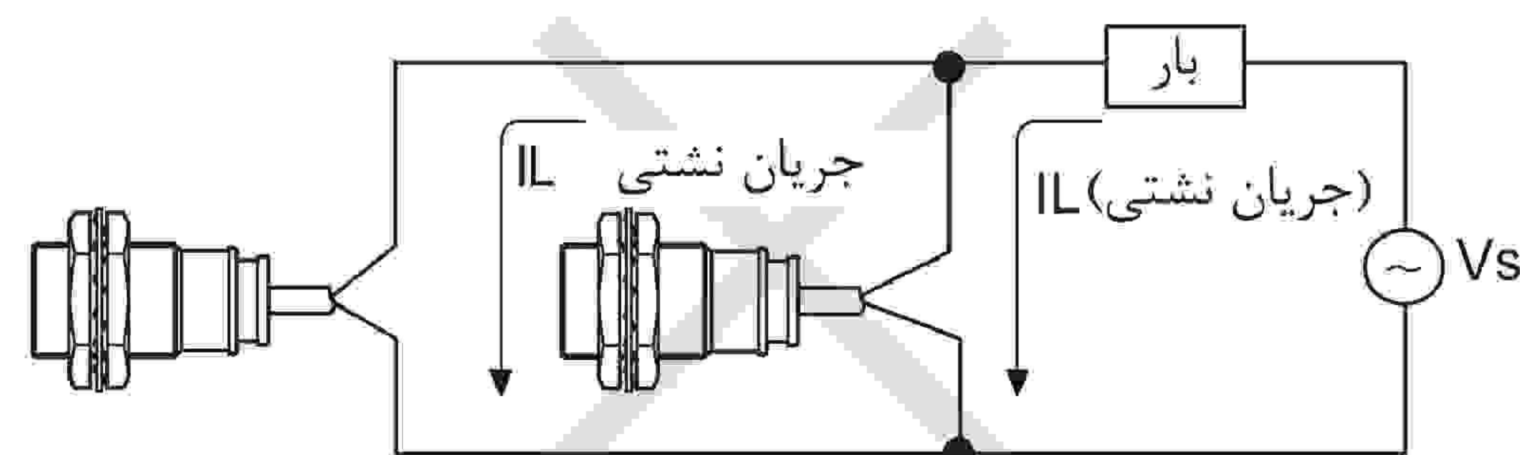
روش نادرست اتصال موازی (شکل ۱)
