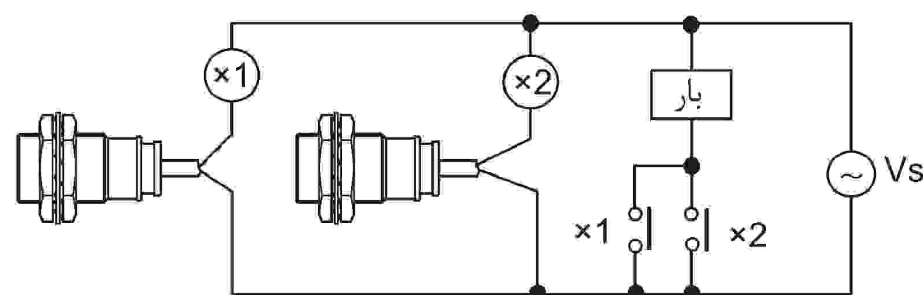
روش صحیح اتصال موازی (شکل ۵)
